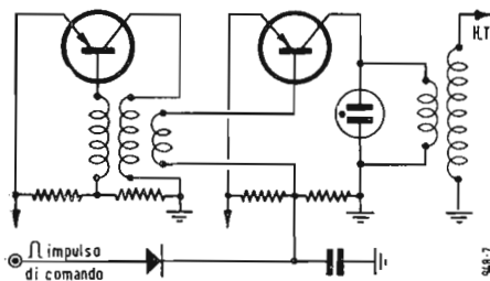
Fig. 1 - Uno degli ultimi dispositivi di accensione elettronica sperimentati: un transistor pilota oscilla in permanenza; ma il secondo transistor da energia al trasformatore solamente quando è sboccato da un impulso proveniente per esempio dal ruttore. Il tubo al neon limita i picchi di tensione inversa, pericolosi per il transistor.
