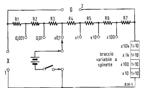
Fig. 3 - Circuito adottato.
