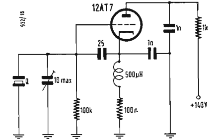
Fig. 8 - Oscillatore di taratura per 10 ÷ 20 MHz.
