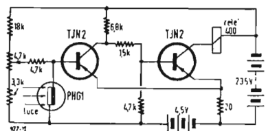
Fig. 3 - Applicazione al circuito di figura 1 per l'azionamento di un relais attraverso un fotodiado.
