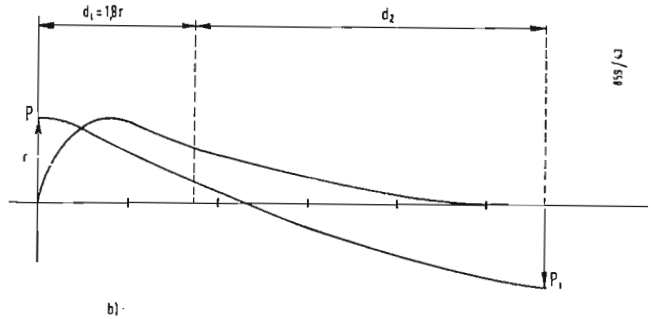
Fig. 26 - Lente catodica: a) Distribuzione del potenziale e delle sue due prime derivate; b) Due traiettorie elettroniche.
