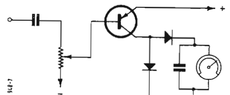
Fig. 3. - Il tachimetro comprende un transistor limitatore d'ampiezza, seguito da un contatore di impulsi ridotto alla sua espressione più semplice. L'alimentazione è fornita da un piccolo alternatore oppure dal circuito di accensione.
