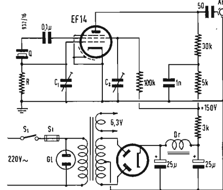
Fig. 6 - Oscillatore a quarzo per 100 kHz ÷ 15 MHz.
