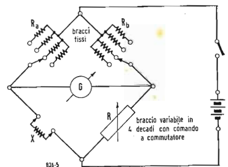
Fig. 1 - Circuito impiegato nei ponti di pregio.
