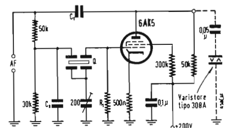
Fig. 2 - Oscillatore a quarzo per 1-10 kHz.
