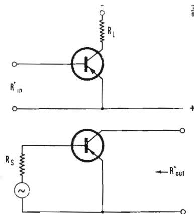
Fig. 3 - Caratteristiche dinamiche, emettitore a massa.
