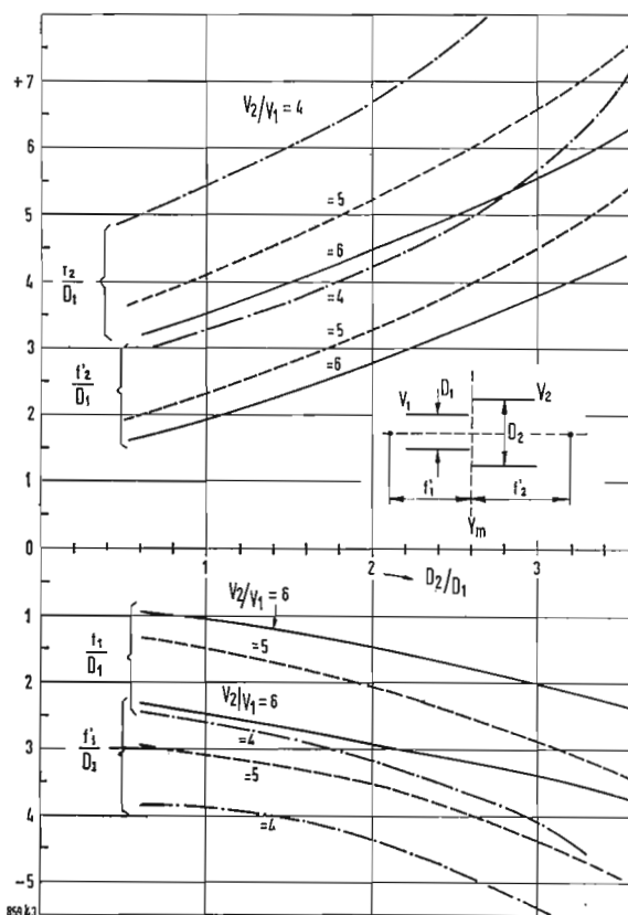
Fig. 22 - Grafici per la determinazione dei punti cardinali della lente elettrostatica a cilindri di diverso diametro.
