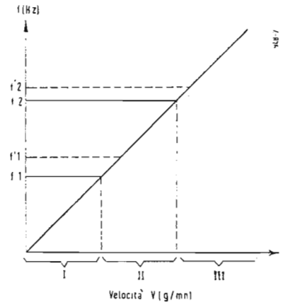
Fig. 5 - Il servomeccanismo provoca normalmente il cambio automatico di velocità per le frequenze f_1 ed f_2 . Se il selettore di marcia è posto nella posizione «sport» il cambio automatico funzionerà alle frequenze f'_1 ( > f_1 ) e ad f'_2 ( > f_2 ).
