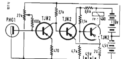
Fig. 4 - Se la variazione di flusso luminoso non raggiunge il valore di almeno 3 millilumen è necessario impiegare uno stadio amplificatore intermedio.
