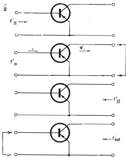
Fig. 2 - Parametri statici del sistema semplificato.
