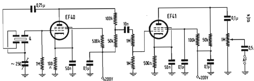
Fig. 1 - Oscillatore a quarzo con stadio disaccoppiatore per 1-60 kHz.
