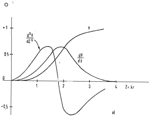
Fig. 26 - Lente catodica: a) Distribuzione del potenziale e delle sue due prime derivate; b) Due traiettorie elettroniche.
