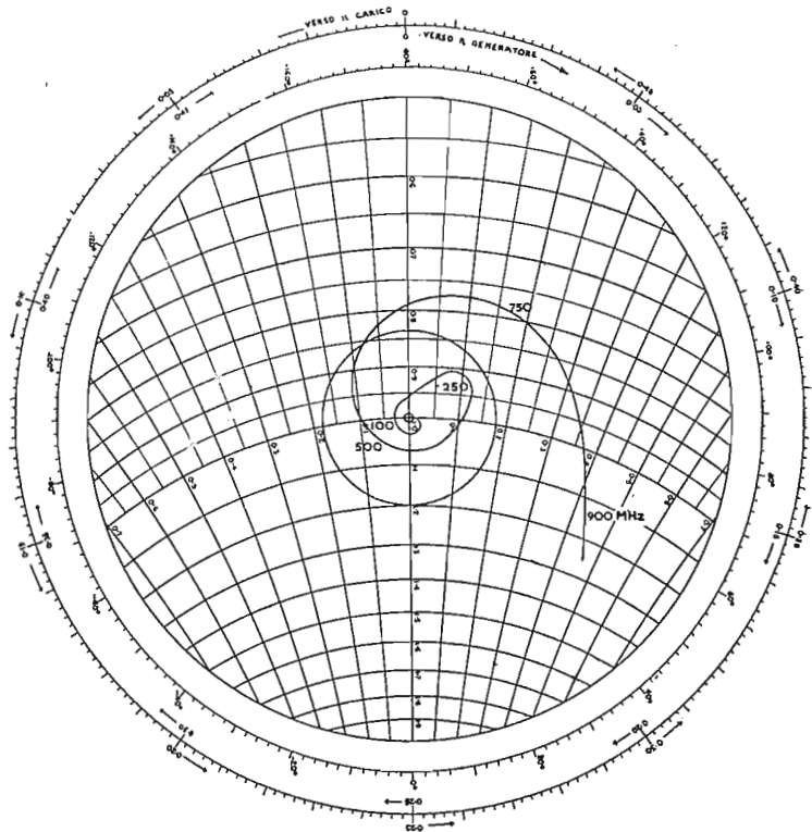
Fig. 6 - Carta di ammettenza del misuratore TF 1152.
