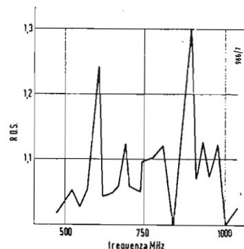
Fig. 5 - Adattamento dei misuratori di potenza.
