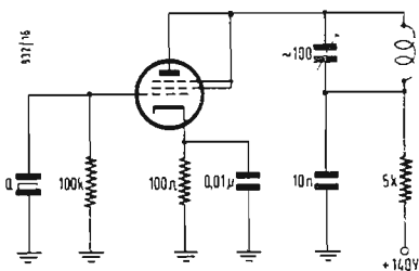
Fig. 9 - Oscillatore di taratura del vobbolatore Grundig 371.
