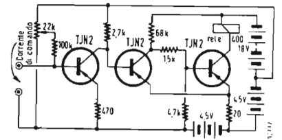
Fig. 2 - Se occorre che la pendolazione del circuito precedente non abbia nessuna ripercussione sui circuiti di comando si potrà aggiungere uno stadio preamplificatore avente nel contempo la funzione di separatore.
